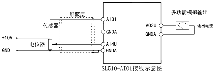
SL510-AIO1接线示意图
